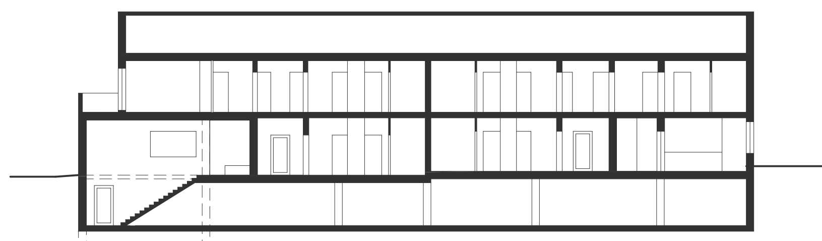
ŘEZ PODÉLNÝ
